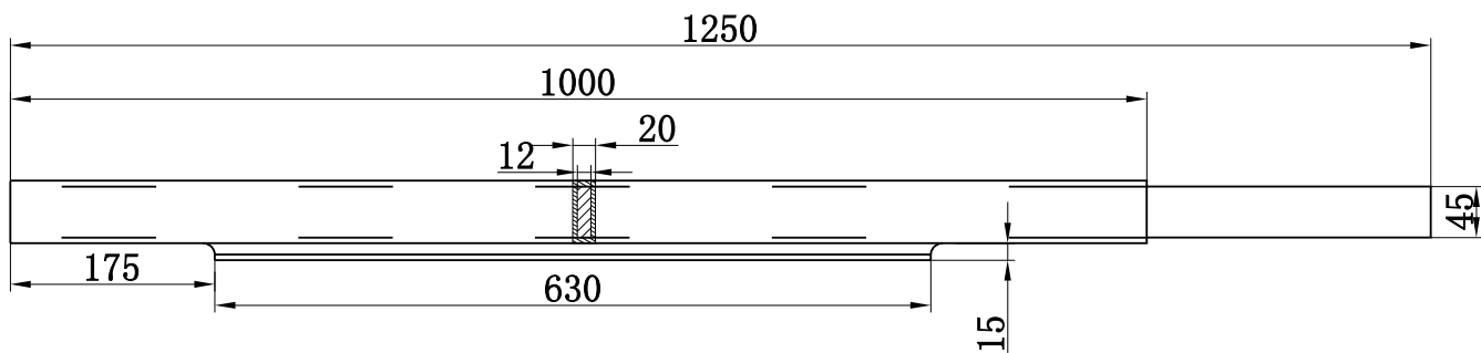
边槽导电棒，主板尺寸同中槽
