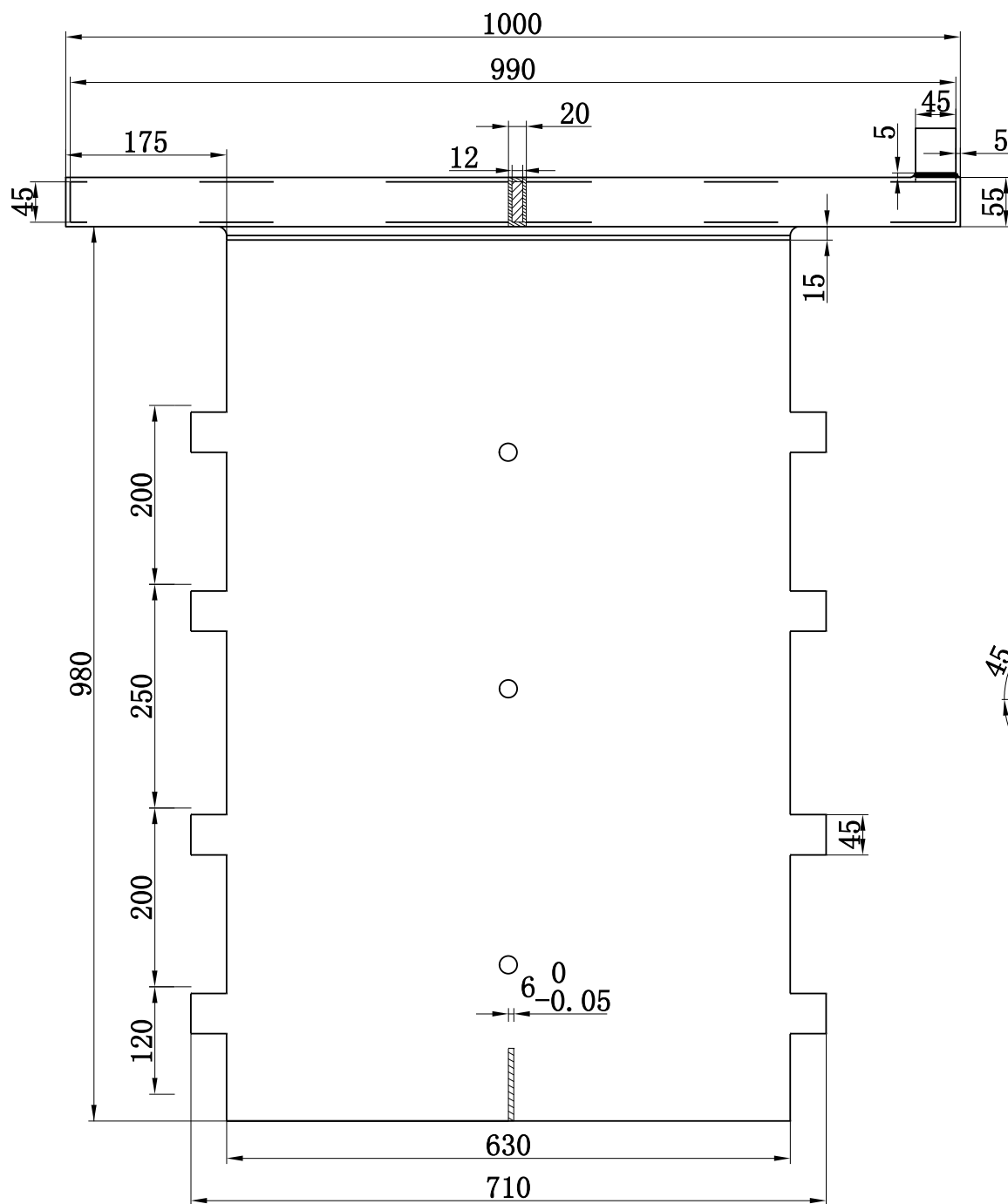
中槽铜头
